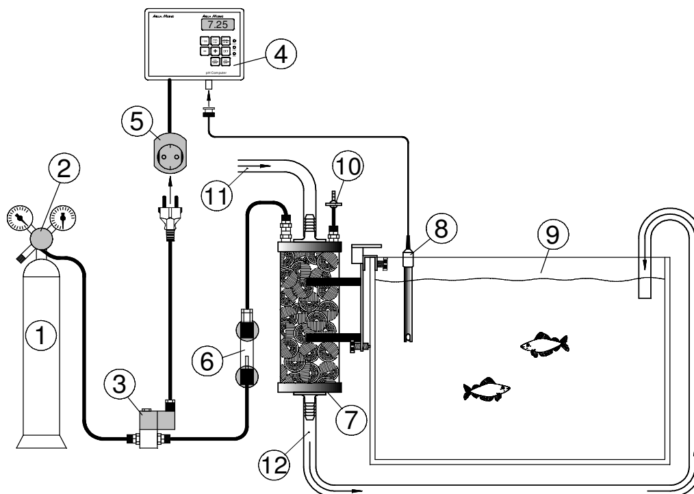
Rys 3: reactor 1000 z automatyczną kontrolą CO 2
